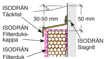
Detalj: Montering ISODRÄN Filterdukskappa.
