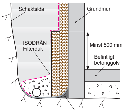
Figur 11. Uppgjutning som tätas med gummiasfalt som stryks på berget, över cementbruksavjämningen och 50-100 mm upp på väggen.
