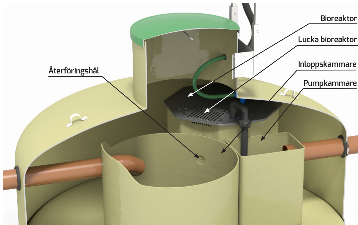
Bild 2. Bioreaktor.
