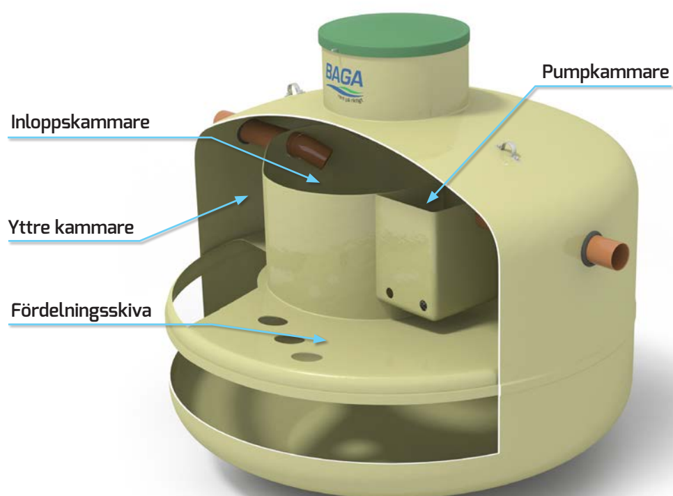
Bild 9. Fördelningsskivan och kamrarna.
